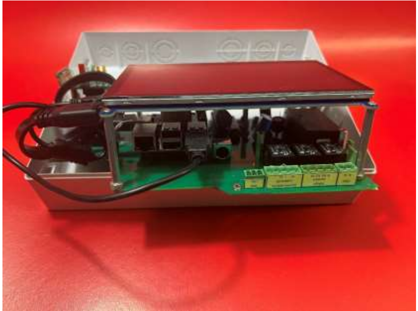
3. kép B61D típusú vezérlőóra csatlakozásainak fényképe
